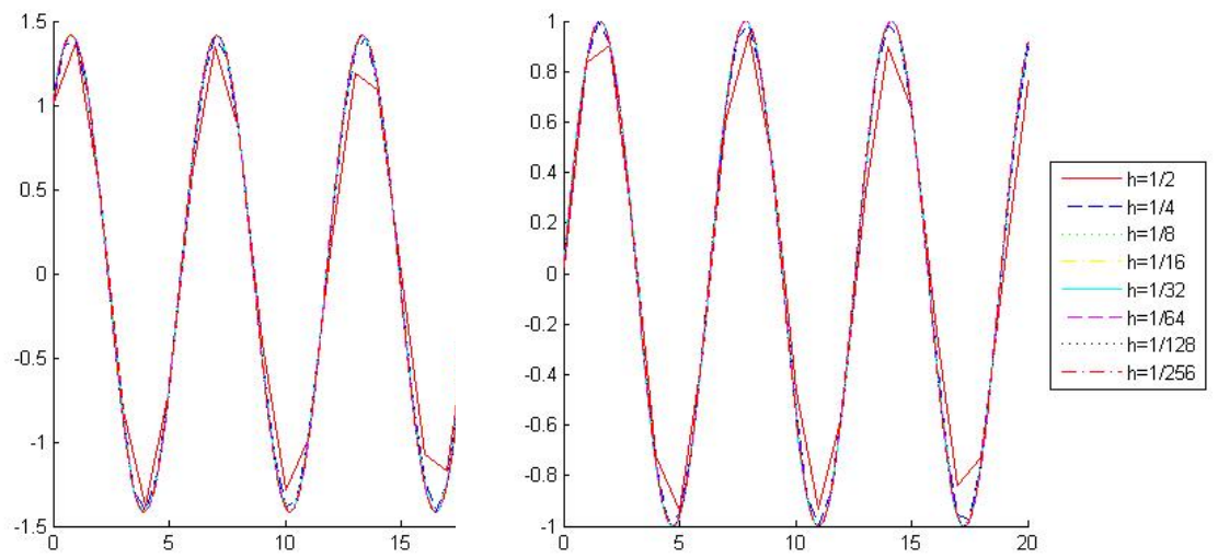
Abbildung 3: klas. Runge-Kutta-Verfahren 1. und 2. Komponente
