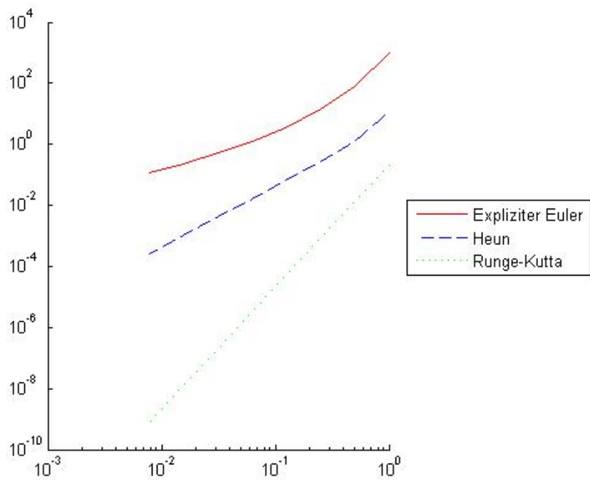
Abbildung 4: globaler Fehler bzgl. der Maximumsnorm
